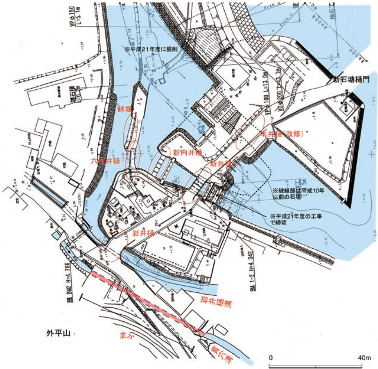
第15図 石塘樋門部分平面図
