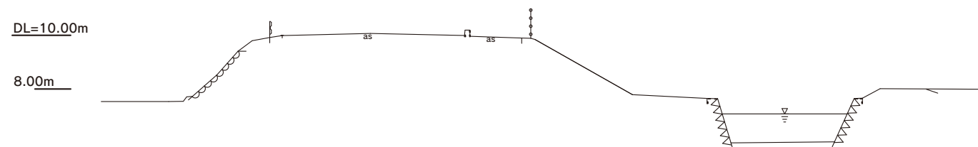
断面図 No.2
