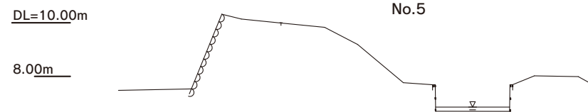
断面図 No.5
