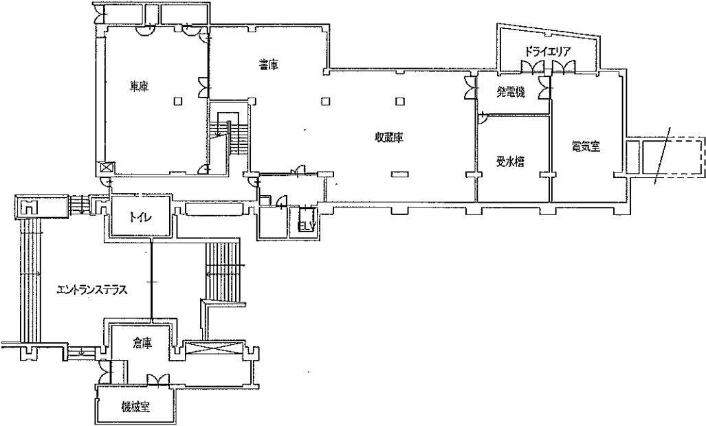
BF平面図 S=1:400
