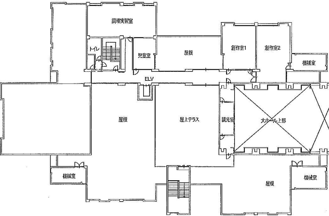
3F平面図 S=1:400
