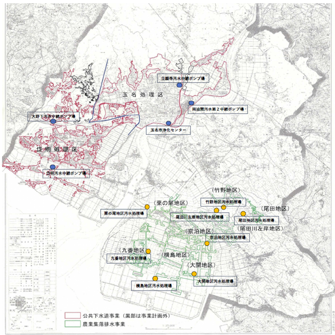
図2 下水道事業施設位置図
