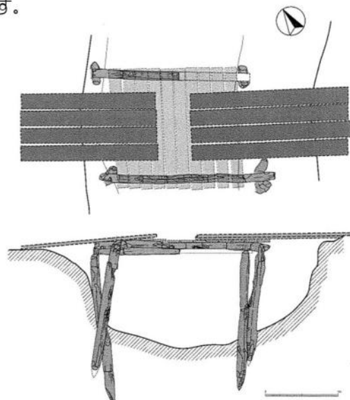
木橋の復元図
