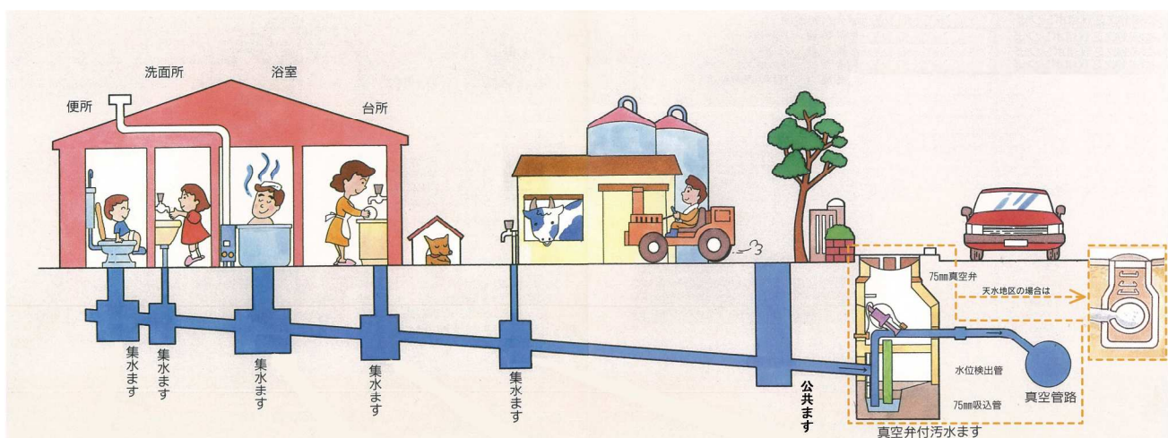
農業集落排水 簡略図
